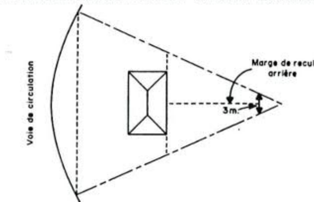
MARGE DE REcul ARRIÈRE POUR LES TERRAINS TRIANGULAIRES
